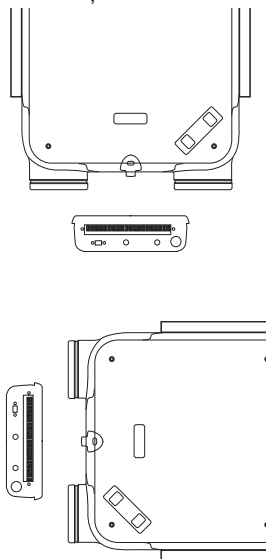
Instalații INCORRECT
