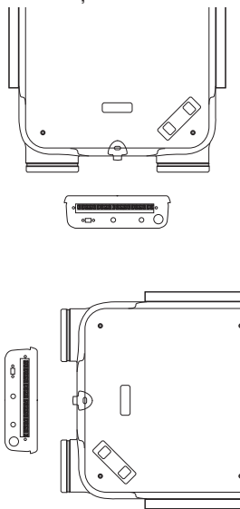
Instalații INCORRECT
