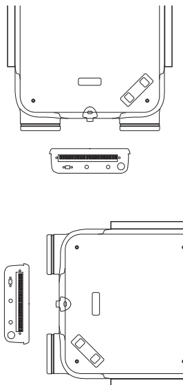
NESPRÁVNÉ instalace
