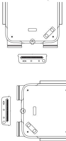
HELYTELEN telepítés
